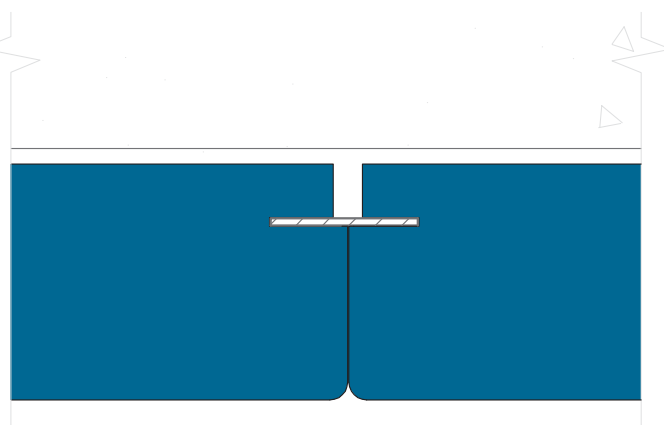
Snittegning av Rockfon VertiQ C i Rockfon System VertiQ C Wall vist med aluminiumsprofiler.
